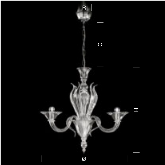
1430/3 Lampadario Ø 72 - H 70 cm R 12,5 cm C 60 cm E14 3x40W 8 kg CE IP20
