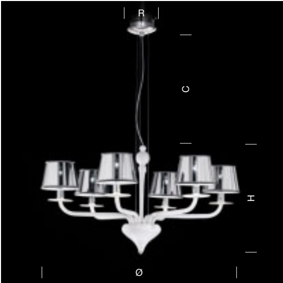
2010/6 Lampadario Ø 92 - H 50 cm R 16,5 cm C 40 cm E14 6x40W 5,5 kg CE IP20
