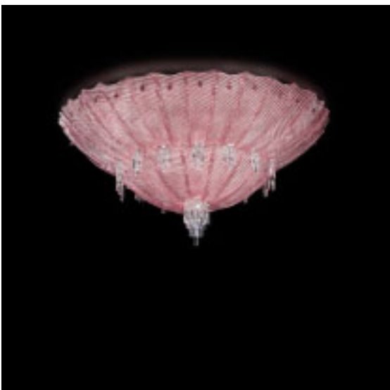
420/110 Plafoniera Ø 110 - H 55 cm E27 12x60W E14 1x60W 55 kg CE IP20
